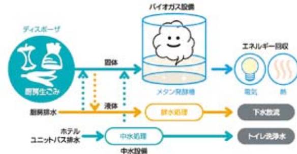
都心型バイオガスシステムの構成
